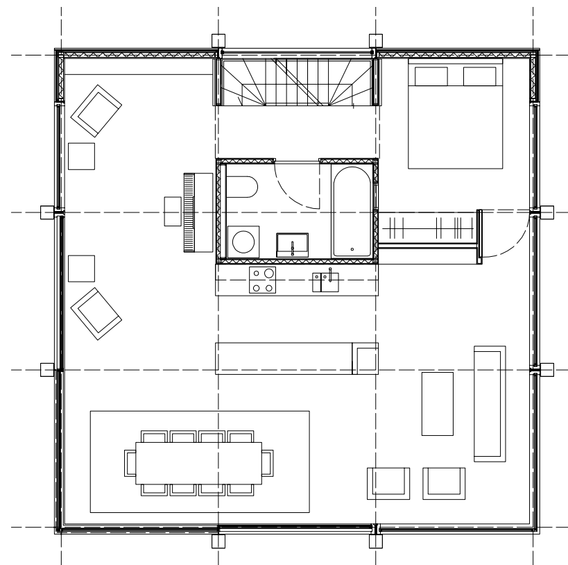
Eerste Verdieping 1:50
