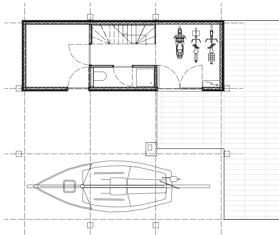
Begane Grond 1:50
