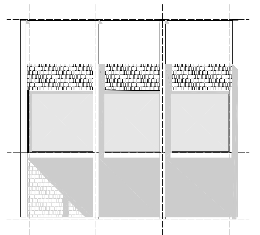
Tweede Verdieping/Dak 1:50
