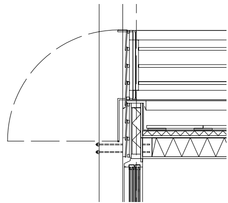
Begane Grond 1:50
