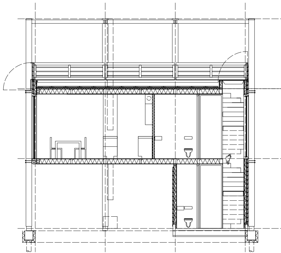
Doorsnede Noord Zuid 1:50
